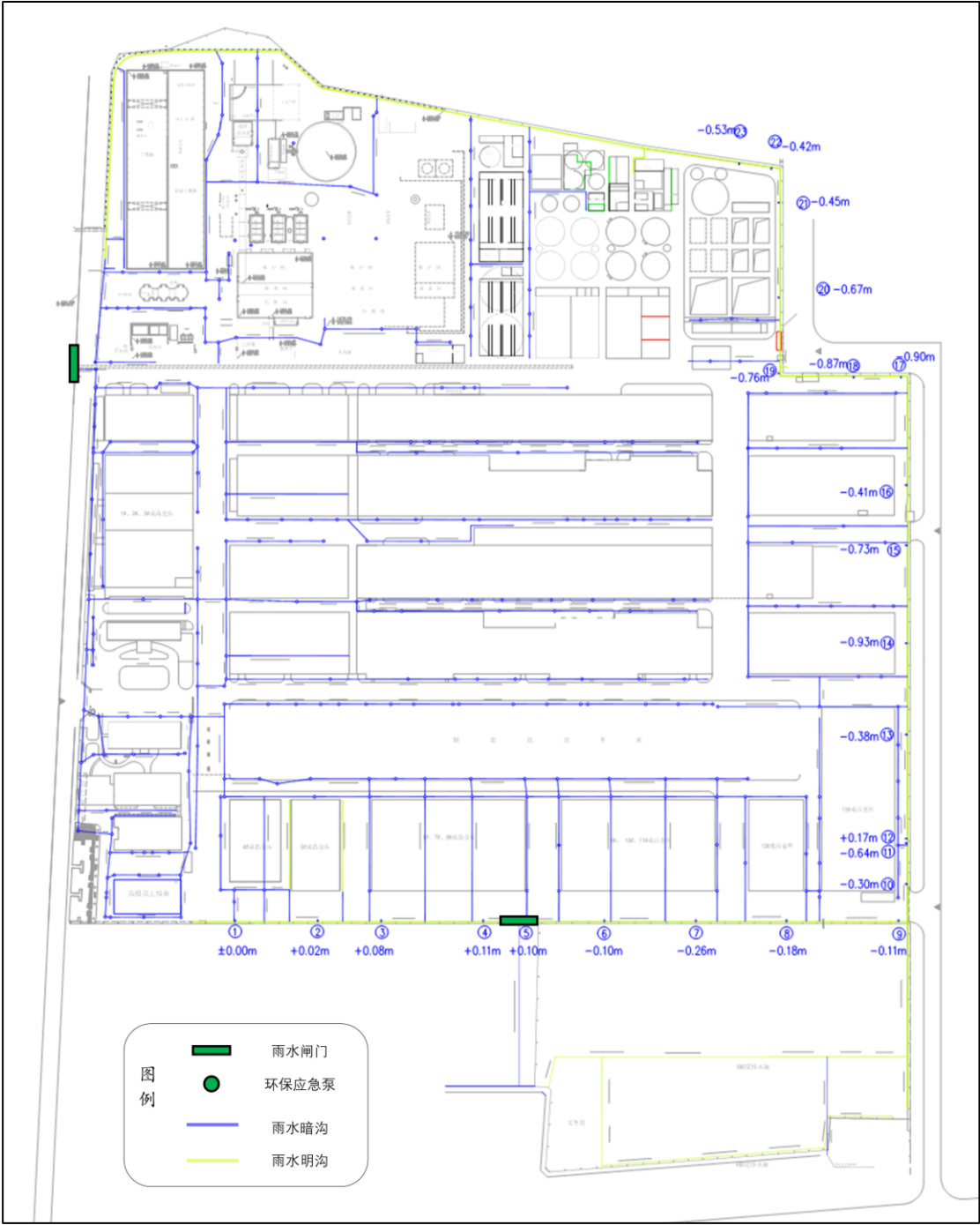
图 6-1 雨水管网图
